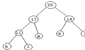
Max-Heap
